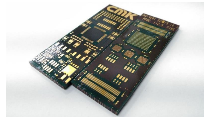
22層(3-16-3) ハイアスペクト基板
